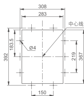
门板开孔尺寸
