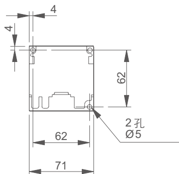
24V外置电源模块
