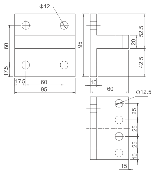
框II A、D、H型断路器T型端子 I_n=800\sim 3200A (最大)
