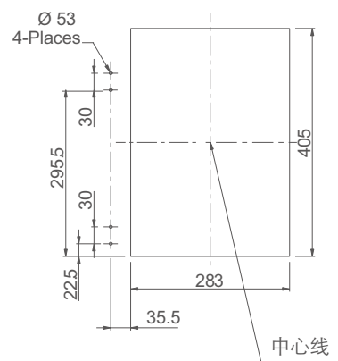
IP54面罩的开孔尺寸
